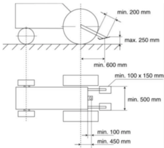
Figuur 1 : Steigerbegrenzer
